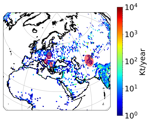
(d) ECLIPSE V6b database SO_2 emissions, 2015
