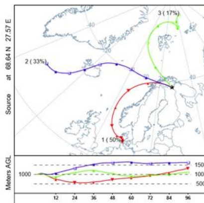
High 7Be values – 20-28/02/2003
