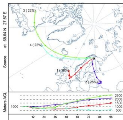
Low 7Be values – 3-16/02/2003
