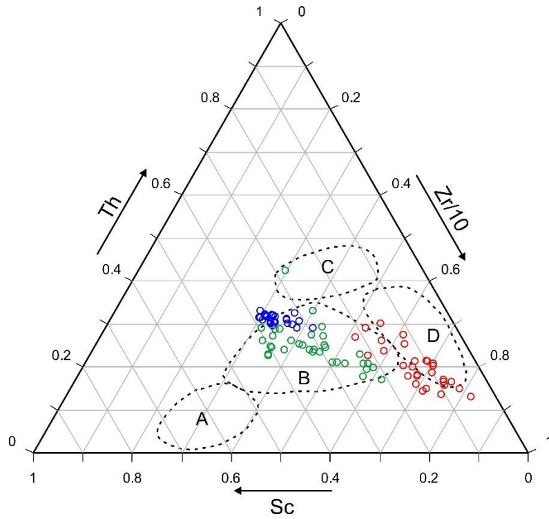
Fig. 2. Th–Sc–Zr/10 plot
