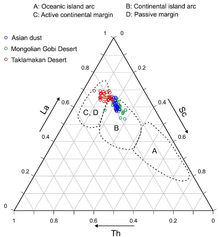
Fig. 1. Th–Sc–La plot
