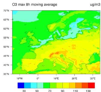
GEM-AQ - spring
