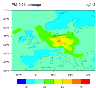
GEM-AQ - autumn
