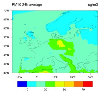
GEM-AQ - summer
