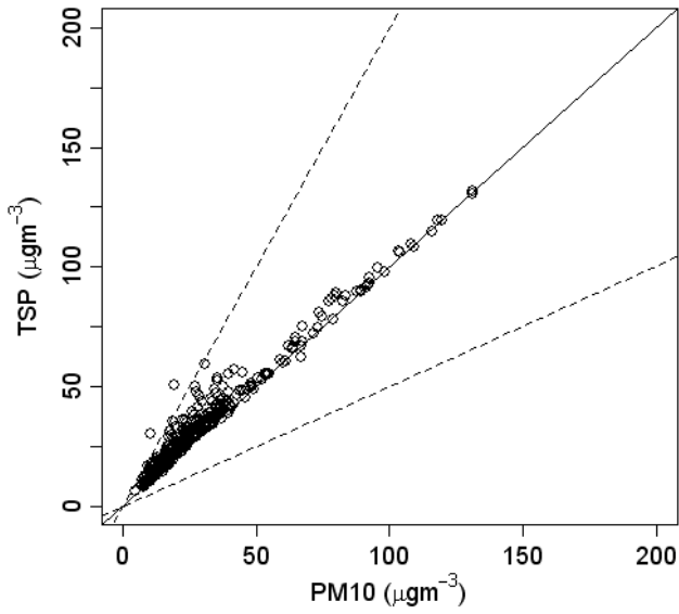
PM10 vs TSP for ZUE
