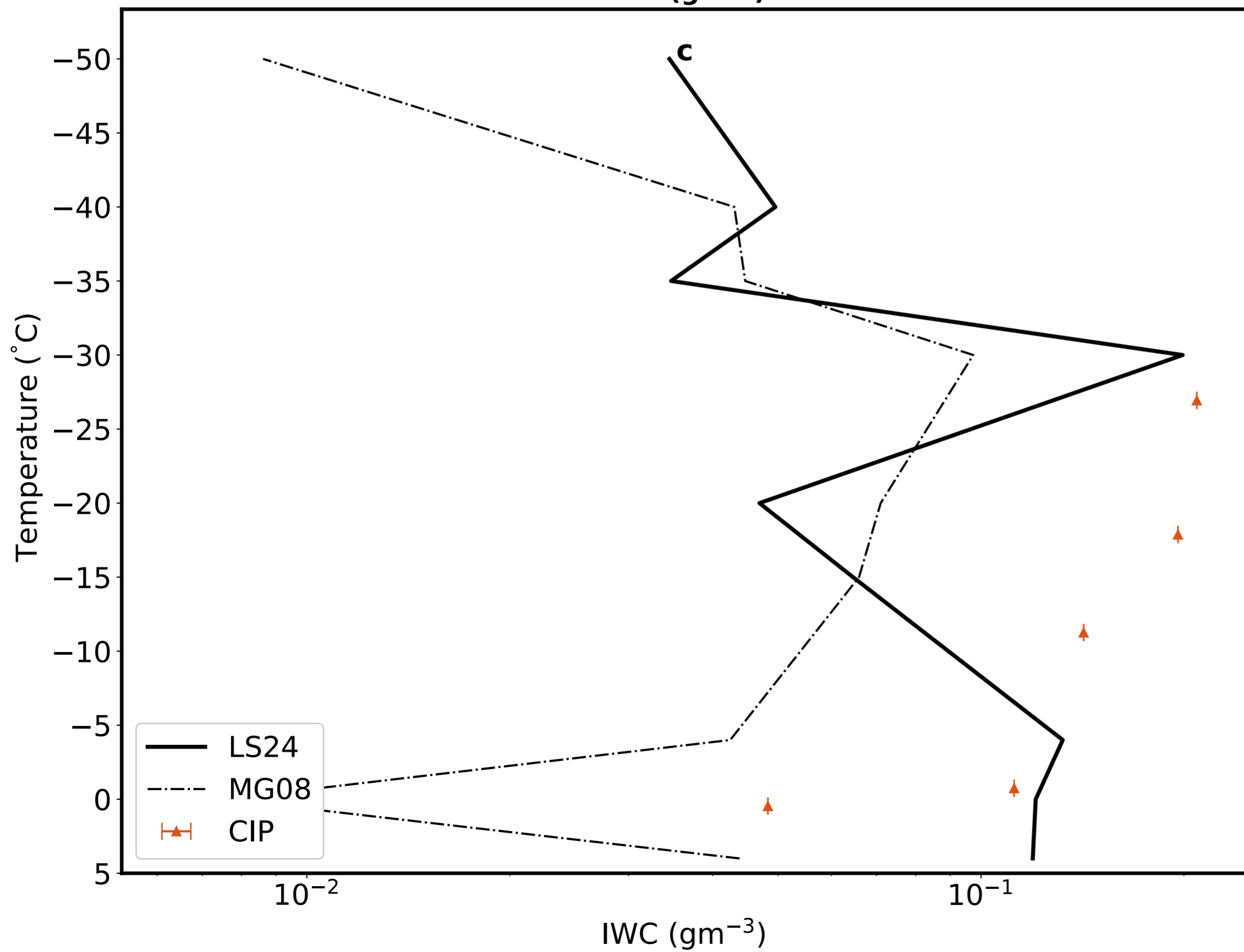
IWC ( gm^{-3} )
