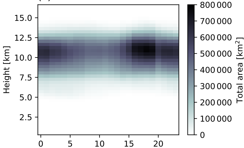
(d) DCC updrafts
