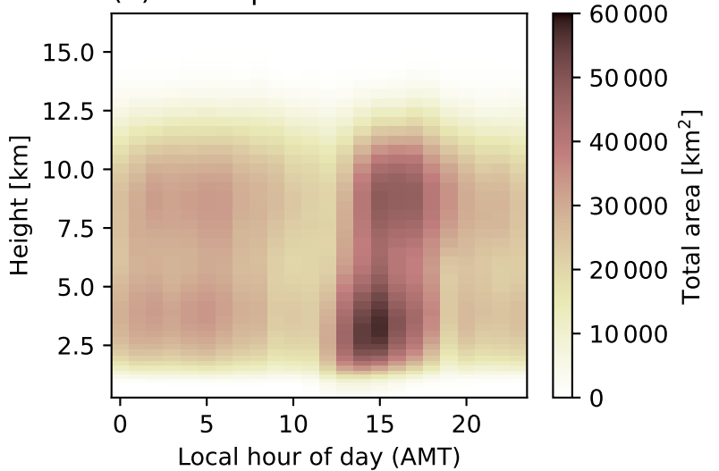
(d) DCC updrafts
