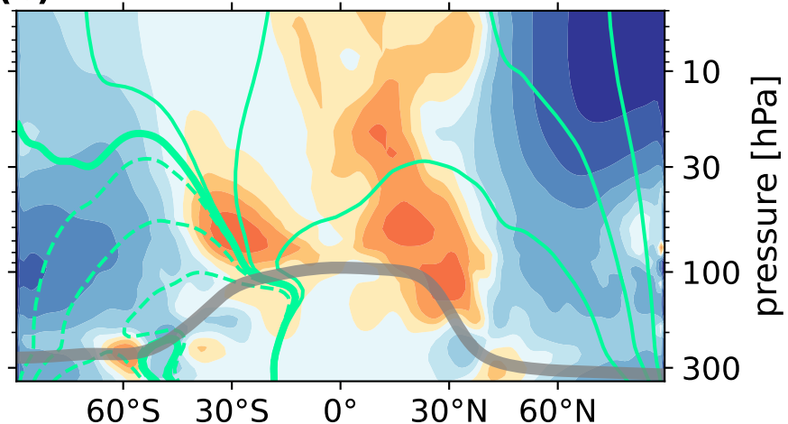
(d) all mixing
