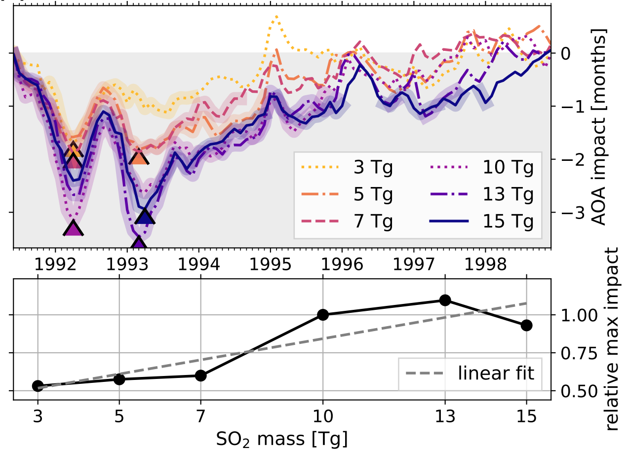
(d) 20N–40N, 30 hPa
