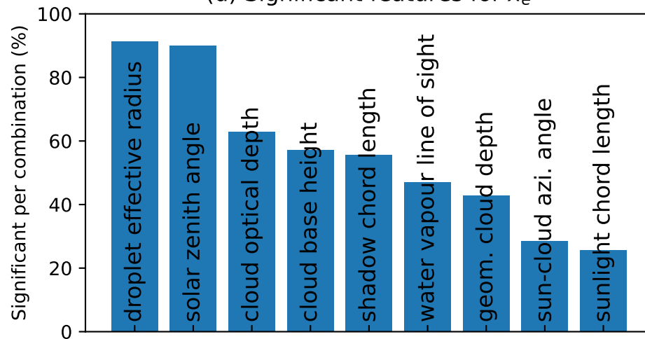
(d) Significant features for x_e
