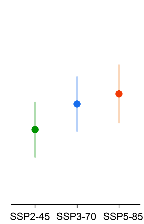
(d) 2091-2100 mean in DJF
