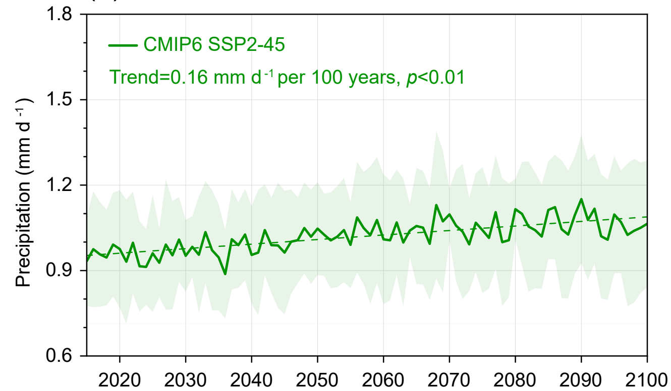
(a) SSP2-45 DJF
