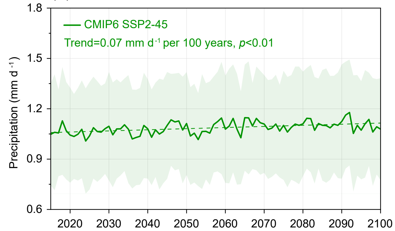
(e) SSP2-45 JJA
