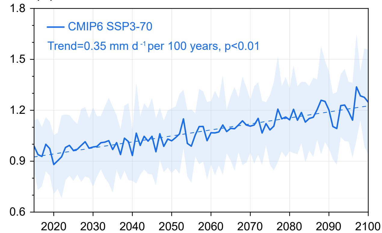
(b) SSP3-70 DJF
