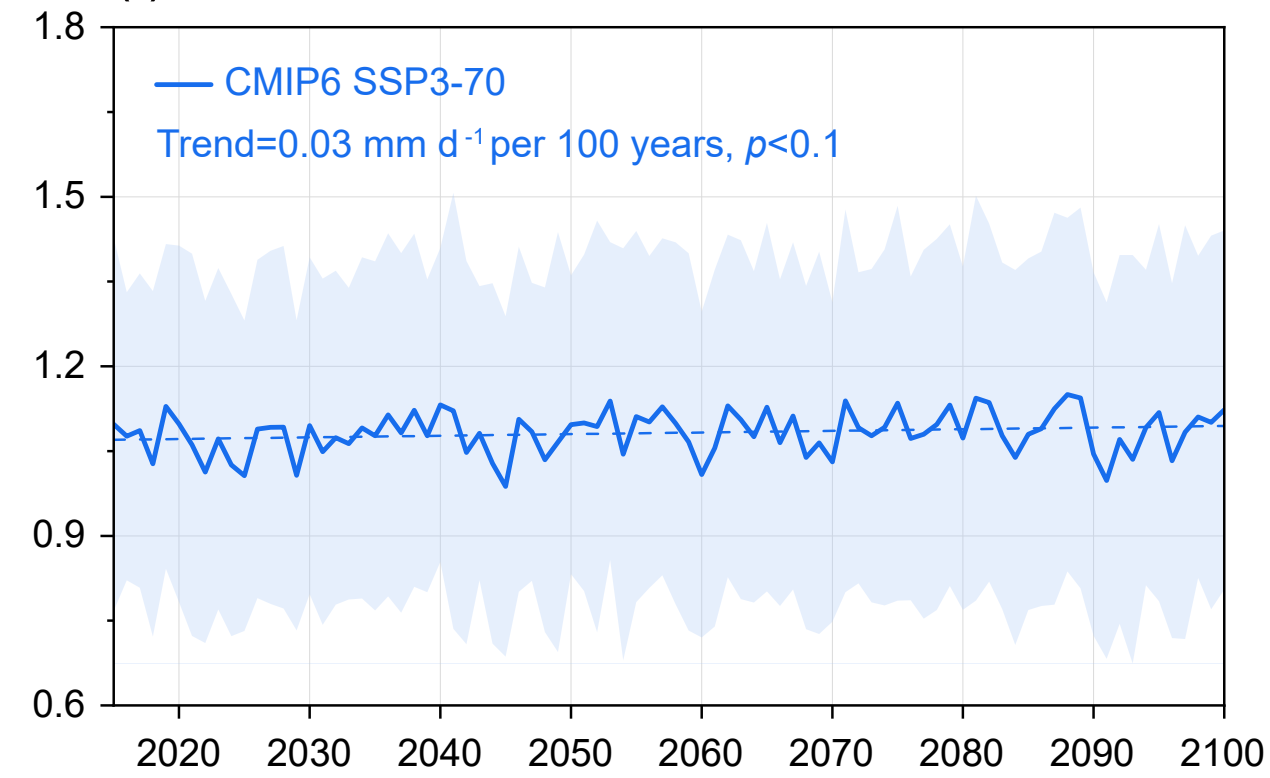
(f) SSP3-70 JJA
