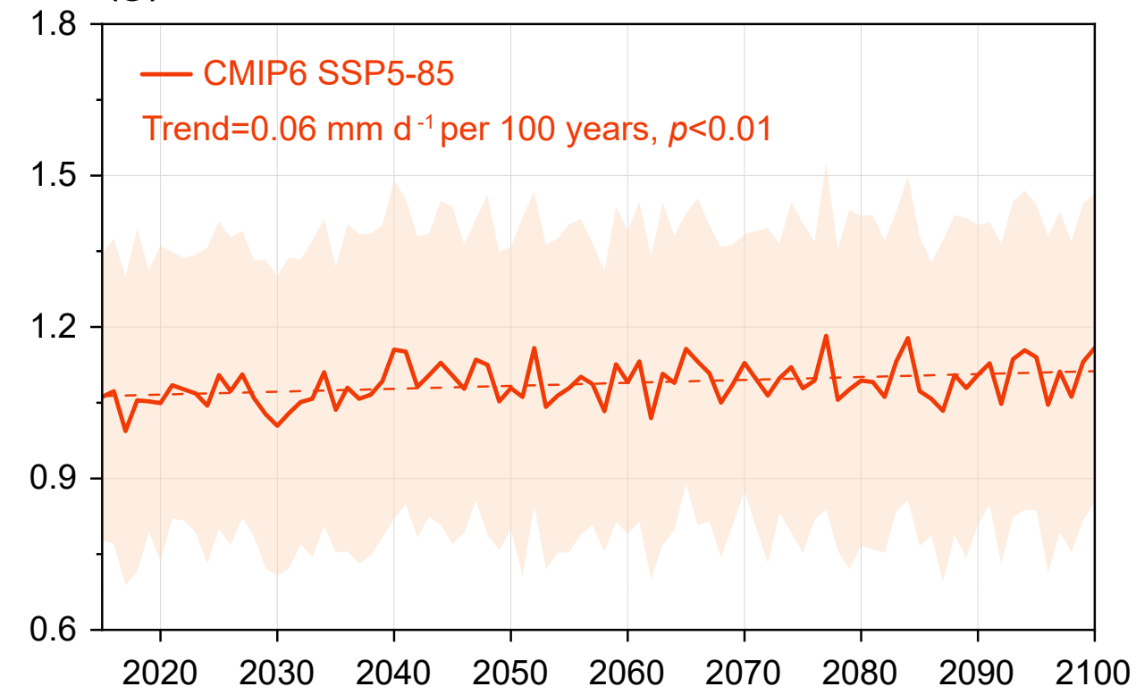
(g) SSP5-85 JJA
