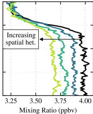
Aerosol \text{SO}_4^{2-}
