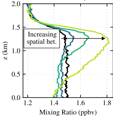
Aerosol \text{NH}_4^+
