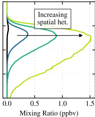
Aerosol \text{NO}_3^-
