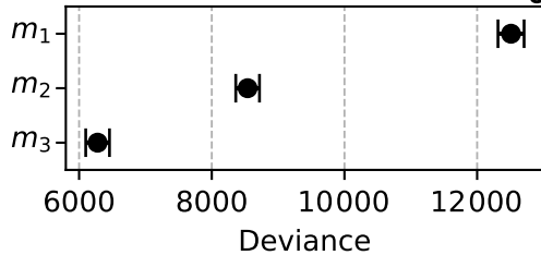
Dataset S_{m_3}
