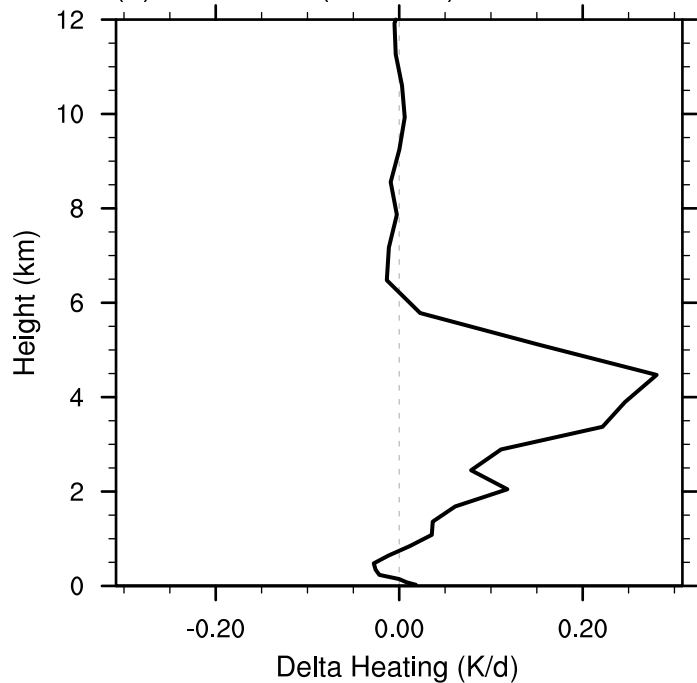
(b) Difference (DA - FR)
