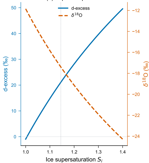
(a) Vapour deposition
