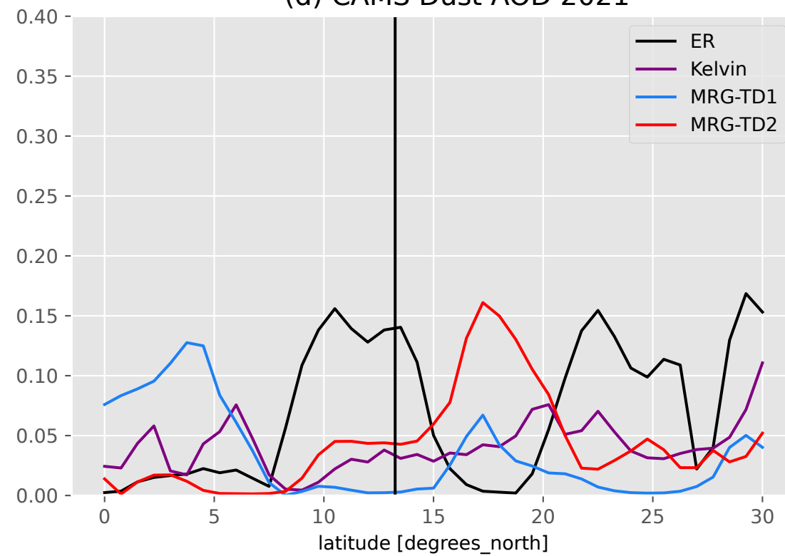
(d) CAMS Dust AOD 2021
