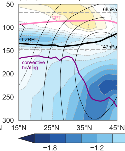
(b) \theta (ERA5-MRM)
