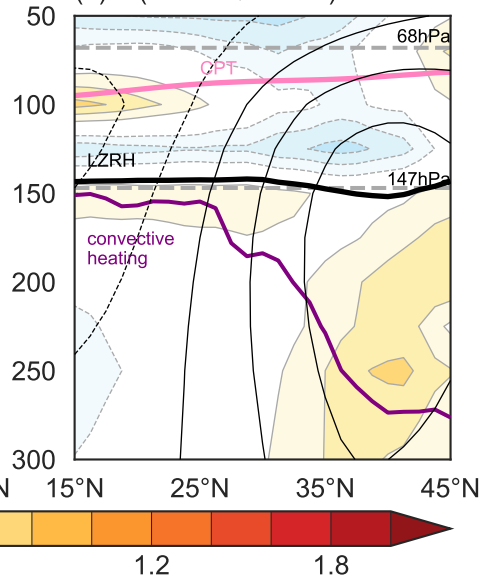
(d) \theta (JRA-3Q-MRM)
