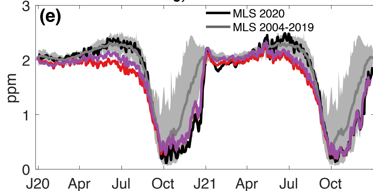
O 3 , 68 hPa
