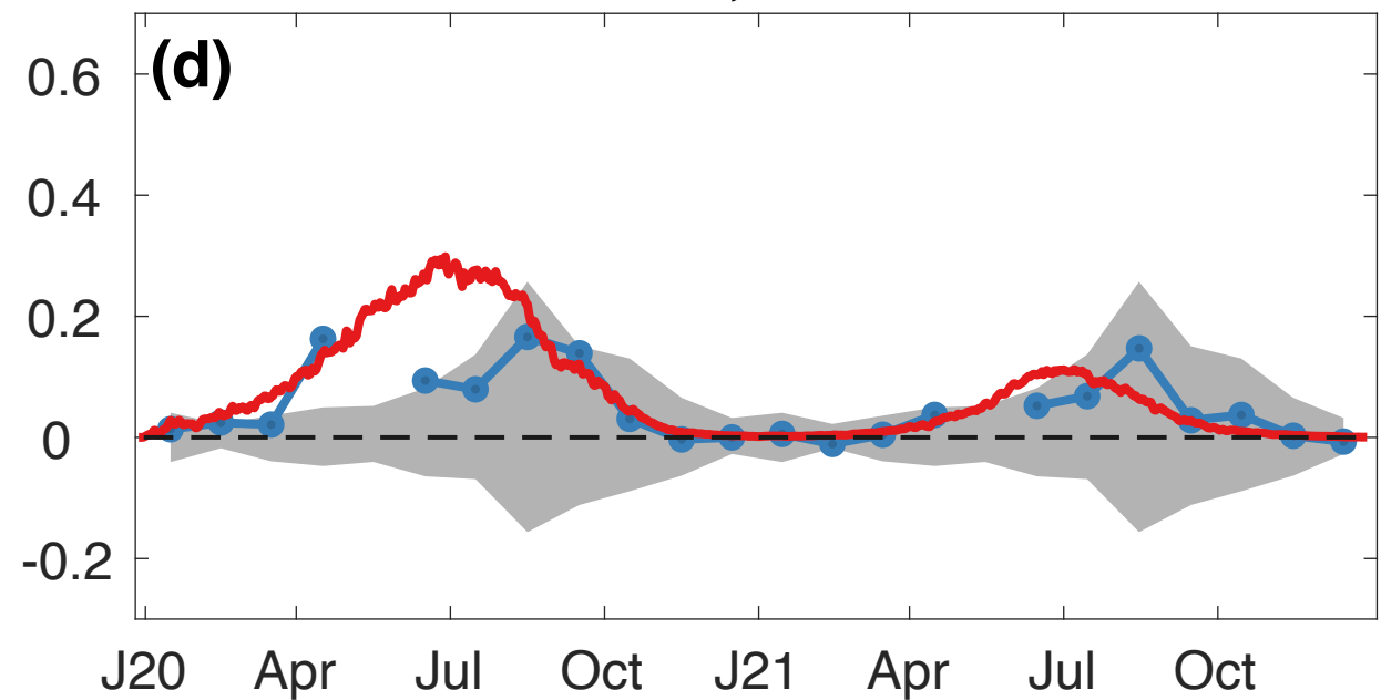
ClO, 100 hPa
