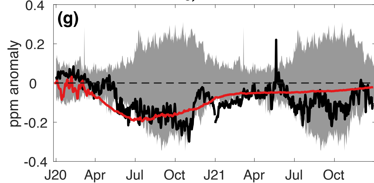
O 3 , 68 hPa
