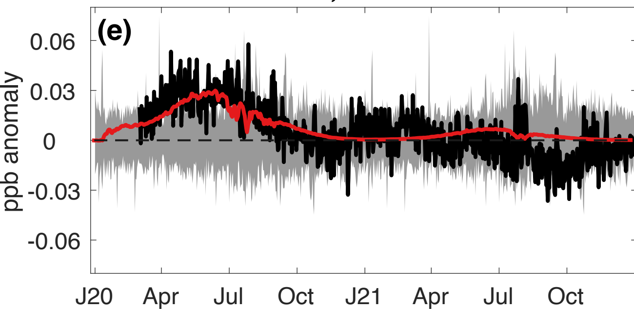
O 3 , 68 hPa
