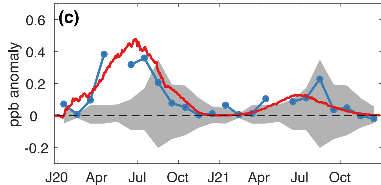
ClO, 68 hPa
