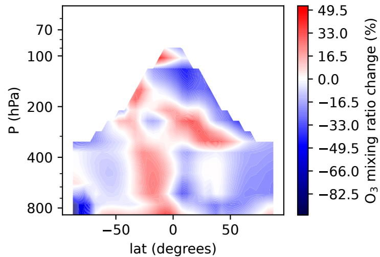
(e) 100 \times (\text{LNOfs}_G - \text{TIER}) / \text{TIER}
