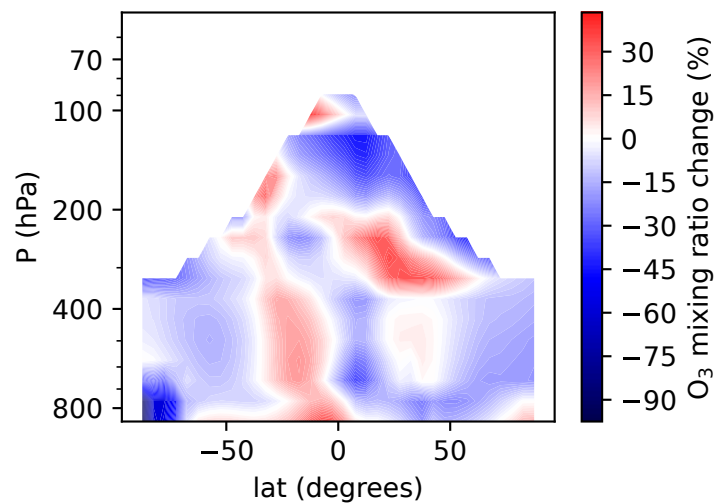
(d) 100 \times (\text{CTR}_G - \text{TIER}) / \text{TIER}
