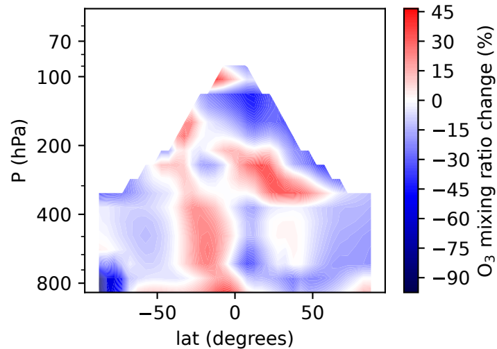
(e) 100 \times (\text{LNOfs}_G - \text{TIER}) / \text{TIER}
