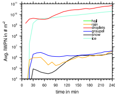
(d) REF: cloud number
