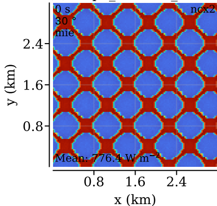
(a) exp3_400m2K_nc
