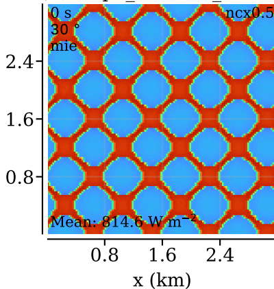
(b) exp3_400m2K_nc
