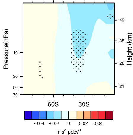
(d) O3 regression U June
