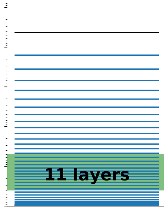
LMDZ-INCA
