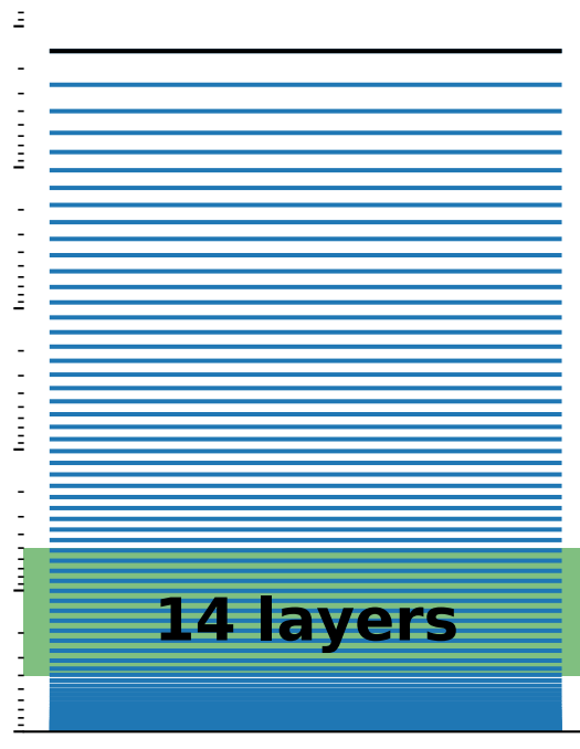
GEOS-Chem
