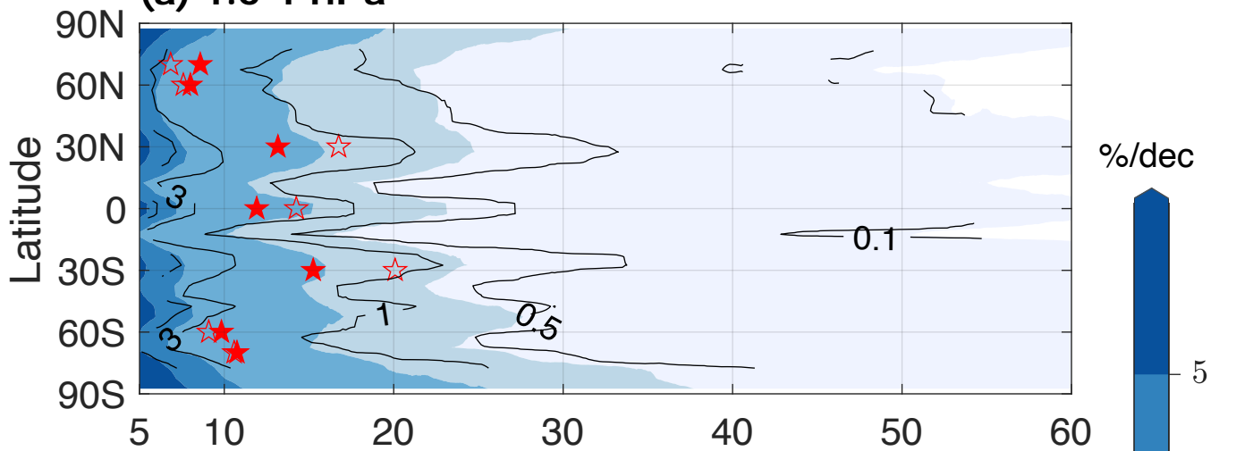
(b) 25-16 hPa
