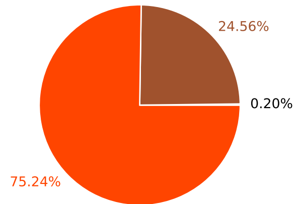
(c) - NOBGSOOT+DUST5
