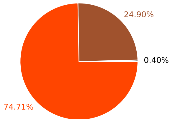
(d) - NOBGSOOT+DUST10
