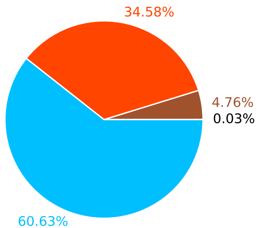
(e) - NOBGSOOT+AMSU
