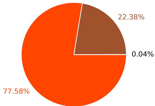
(b) - NOBGSOOT
