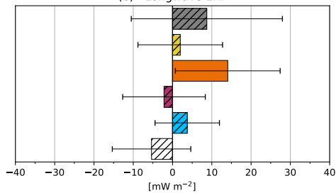
(d) - Longwave ERF (clear-sky)
