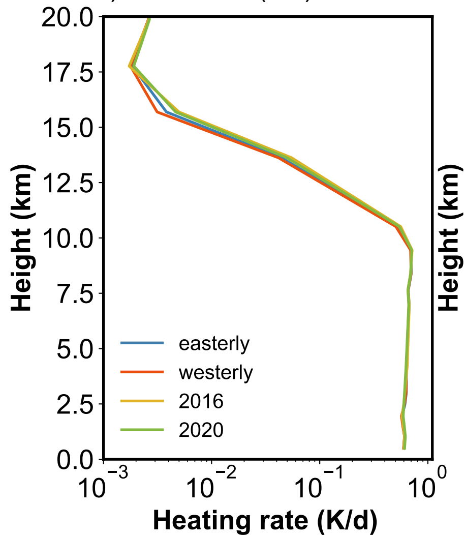
a) H2O DW1 (1,1), MERRA2
