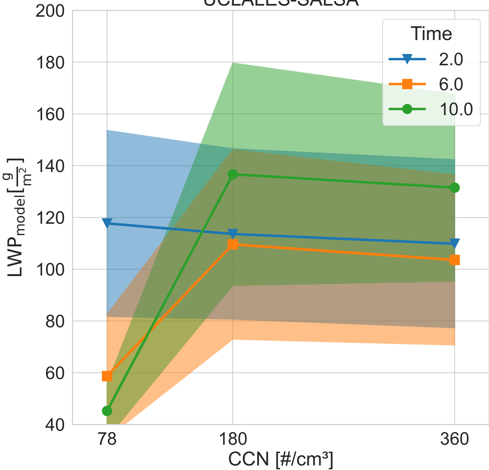
UCLALES-SALSA
