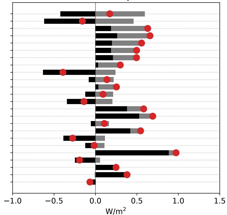
(d) Low Cloud Amount Adjustment
