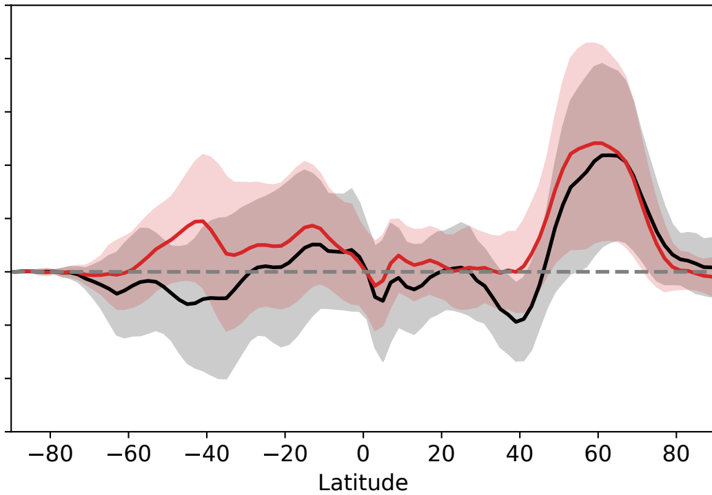
(d) Low Cloud Amount Adjustment
