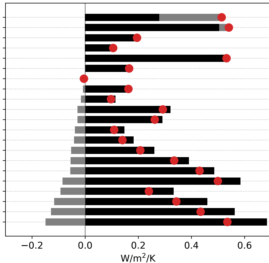
(d) Low Cloud Amount Feedback
