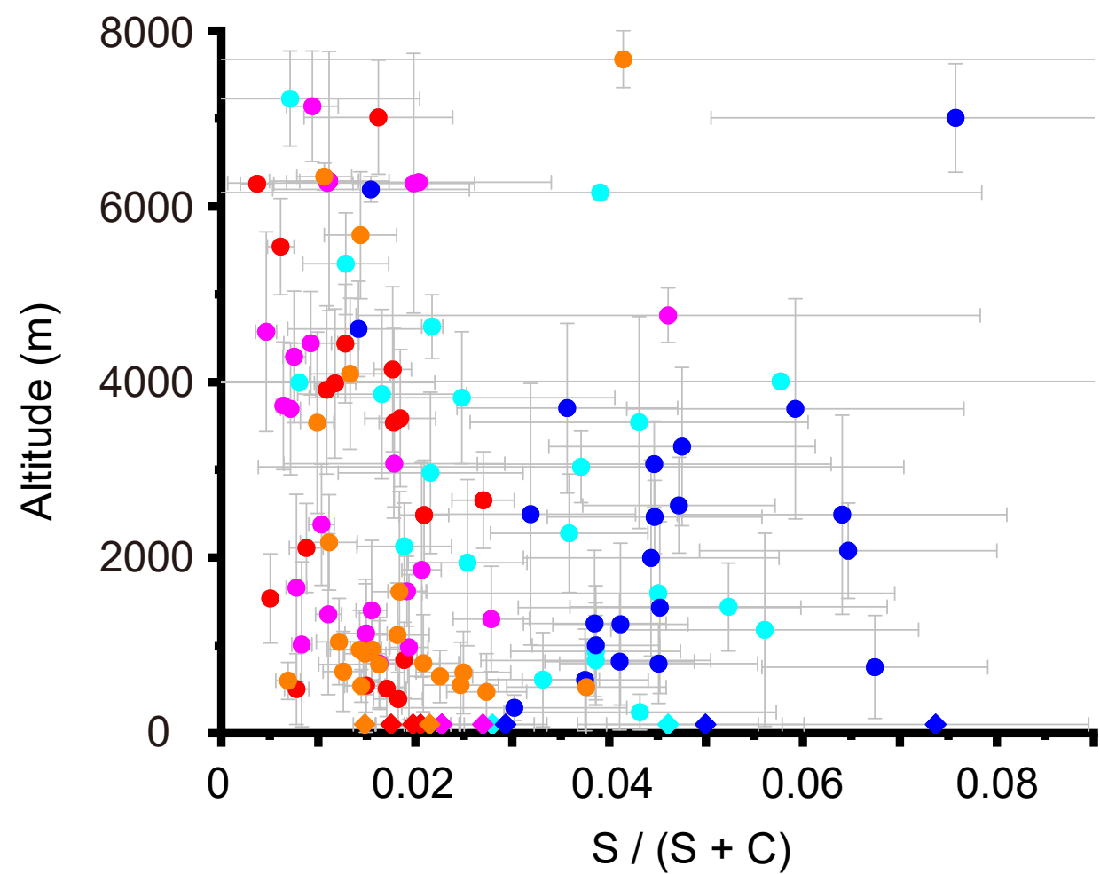
(b) \text{S} / (\text{S} + \text{C})
