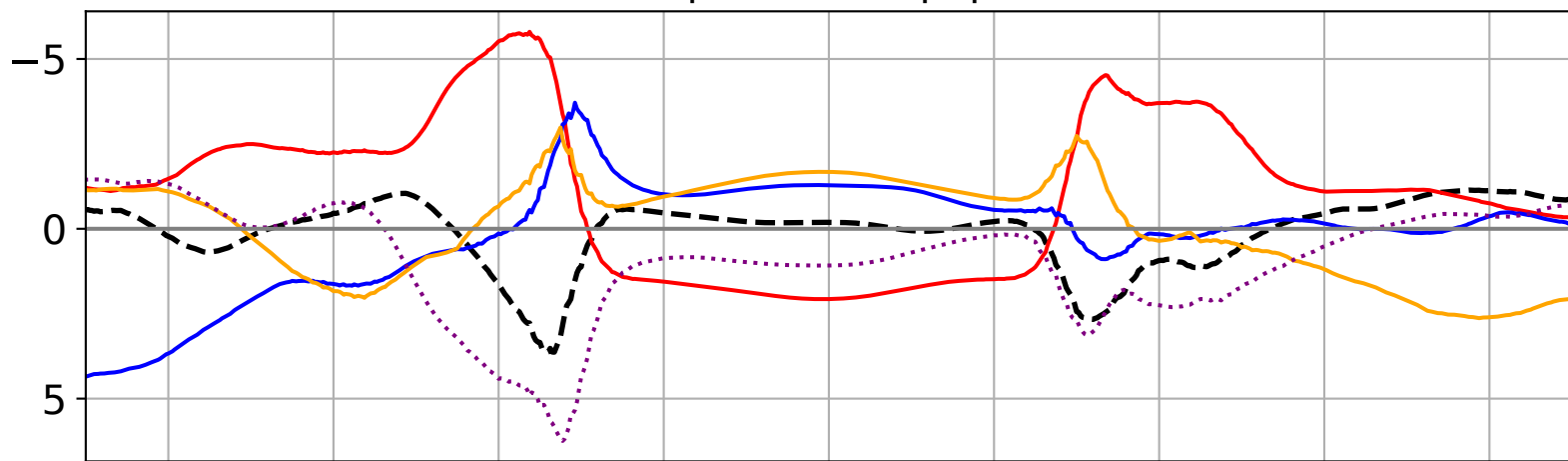
(b) 380 K
