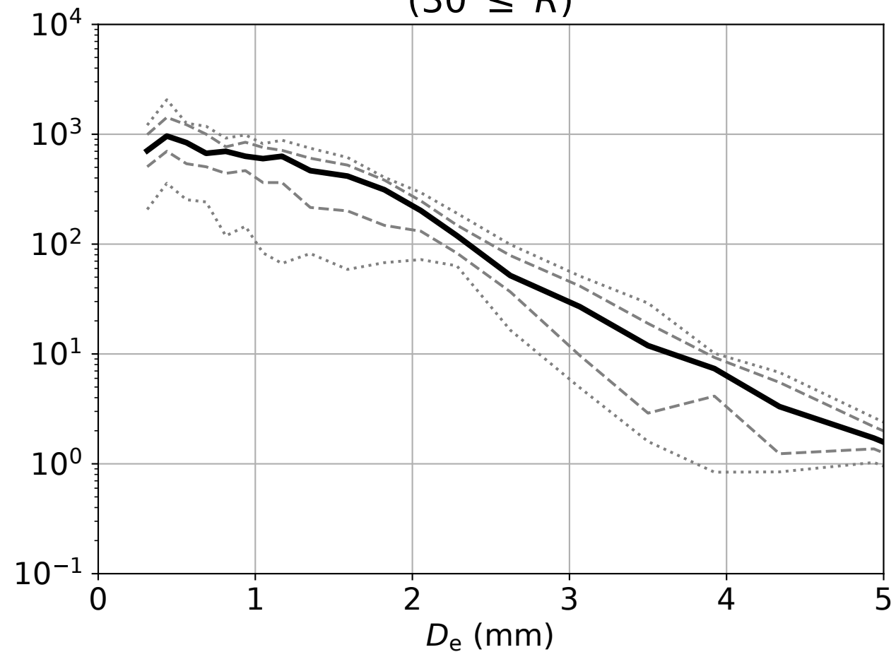
(d) DSD at Kumagaya: # of DSDs = 22 ( 30 \leq R )
