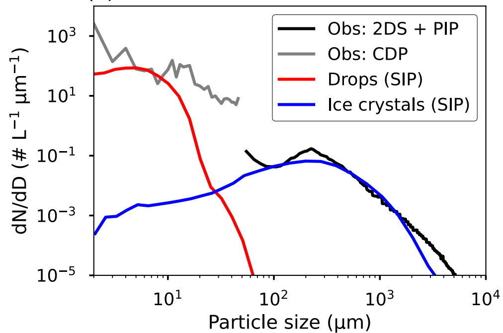
(d) SIP: 7 to 7.5 km
