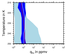
(d) FRZ Ice content
