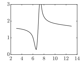
Carbonates: Calcite
