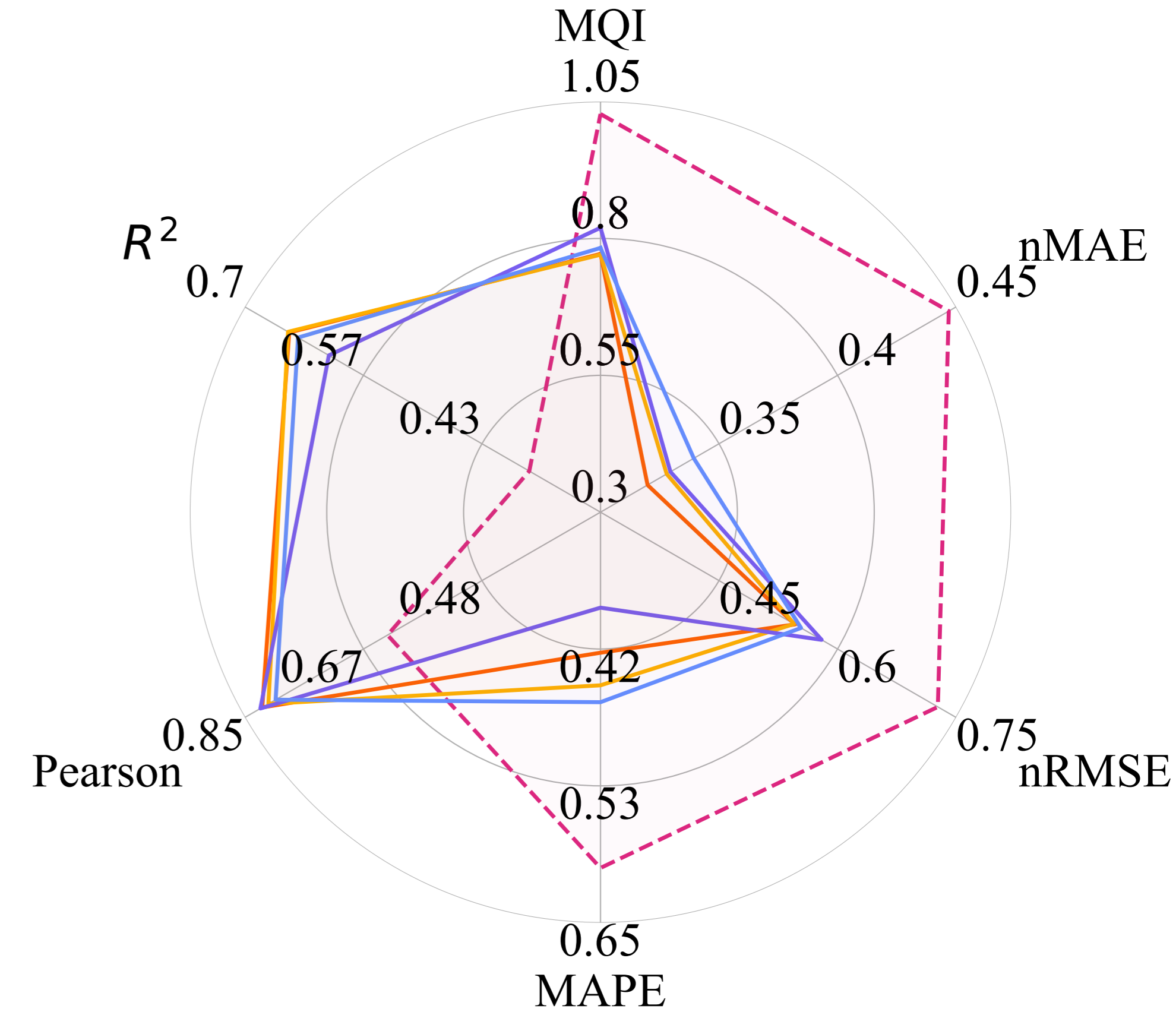
Hornsgatan - NOx
