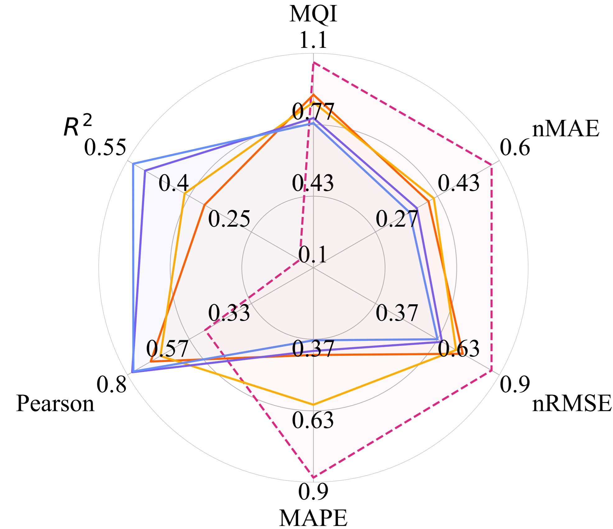
Folkungagatan - NOx
