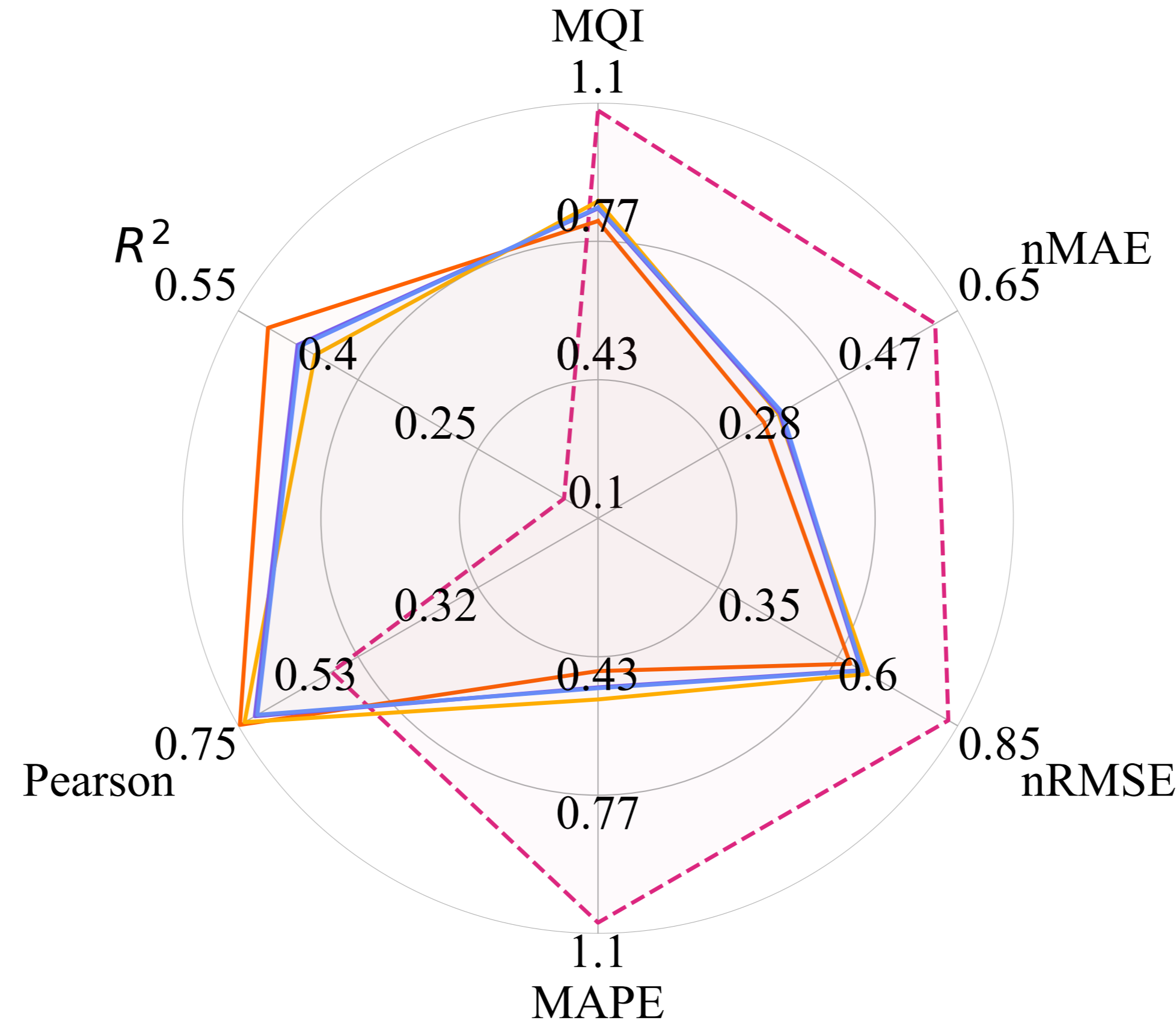
Sveavägen - NOx
