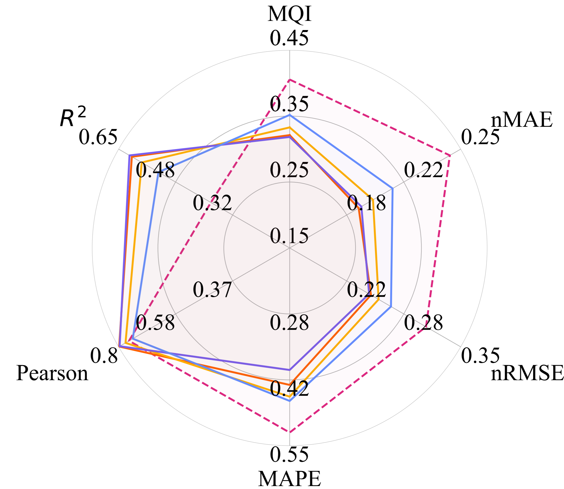
Urban Background - O3
