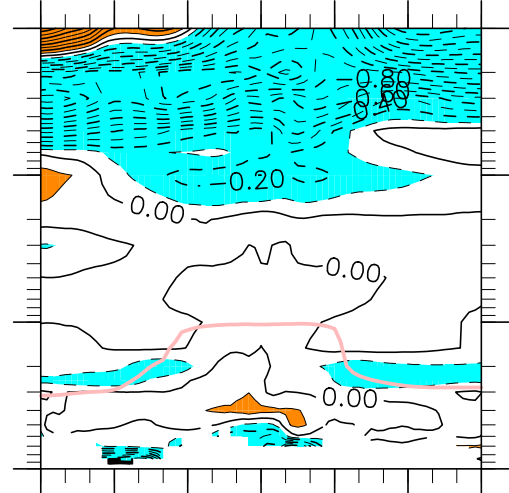
(d) CFSR - REM
