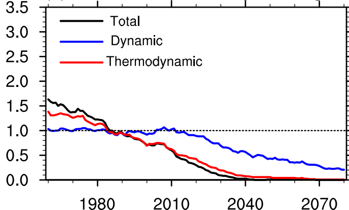
(d) Occurrence probability ratio SAT
