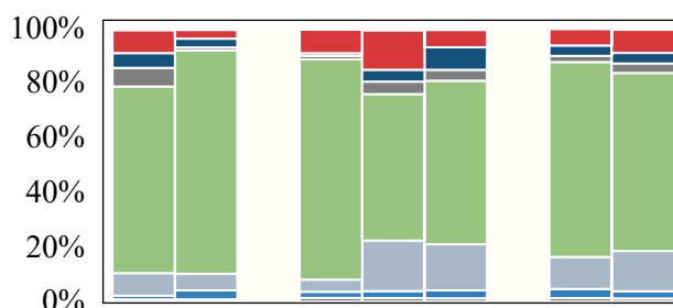
(d) WSOC-CHOS group
