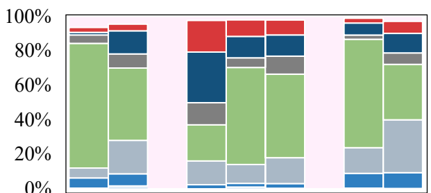
(j) WIOC-CHONS group
