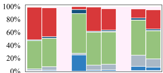
(i) WIOC-CHOS group
