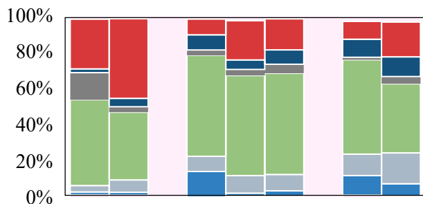
(g) WIOC-CHO group
