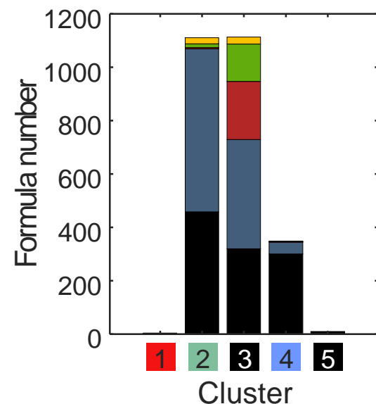
ambient PM (N09)
