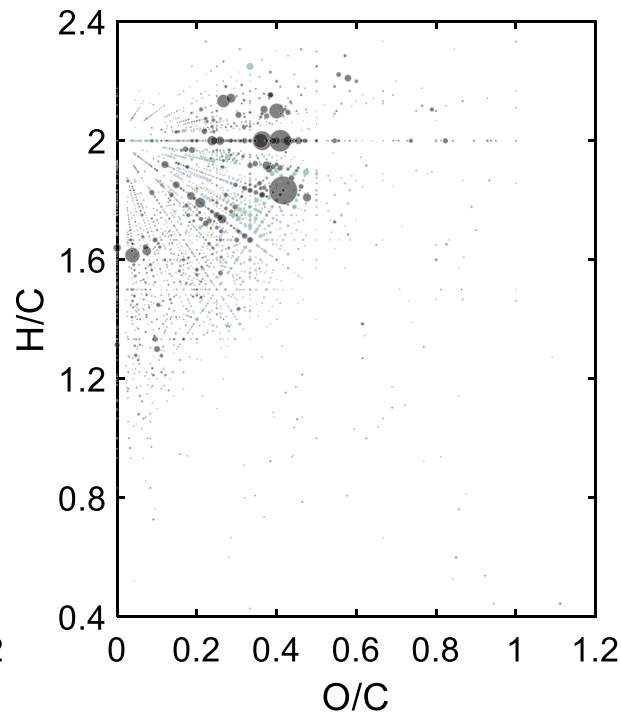
ambient PM (N09)
