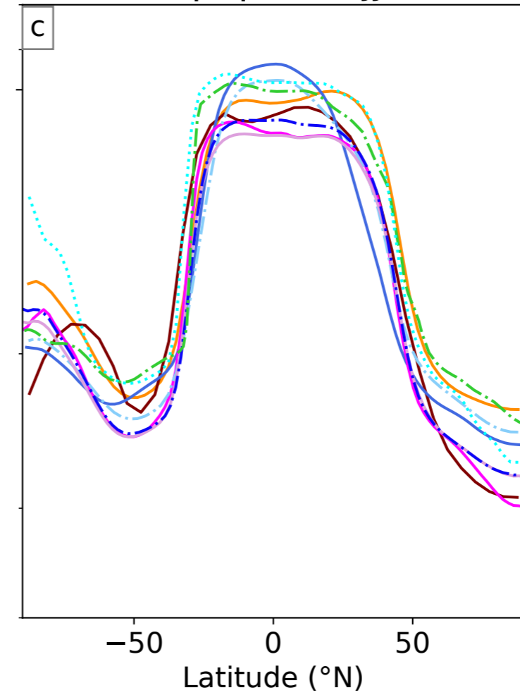
Tropopause JJA
