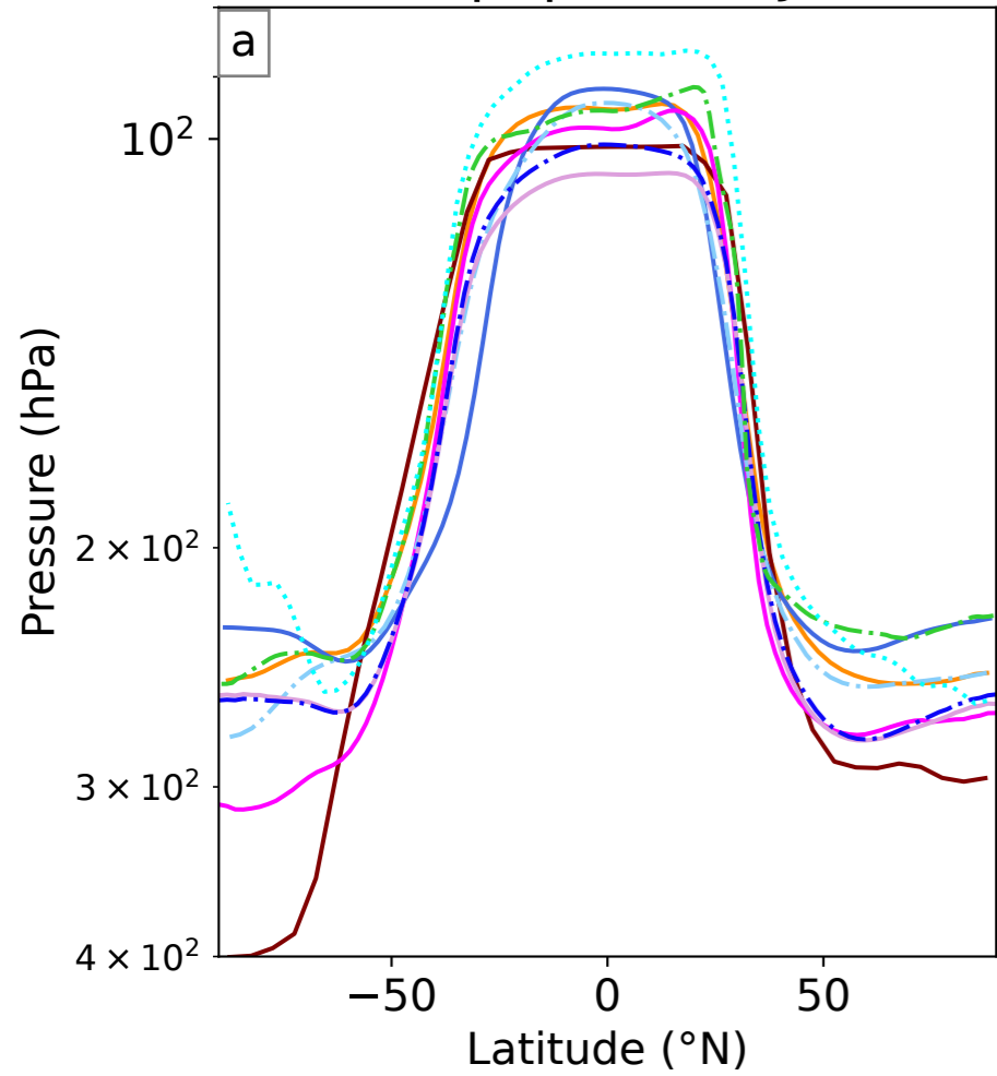
Tropopause DJF
