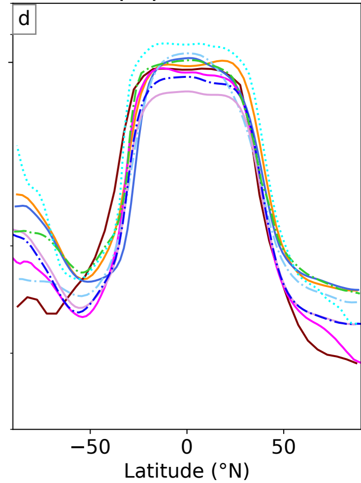
Tropopause SON
