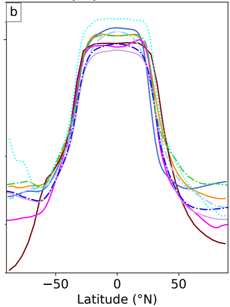
Tropopause MAM
