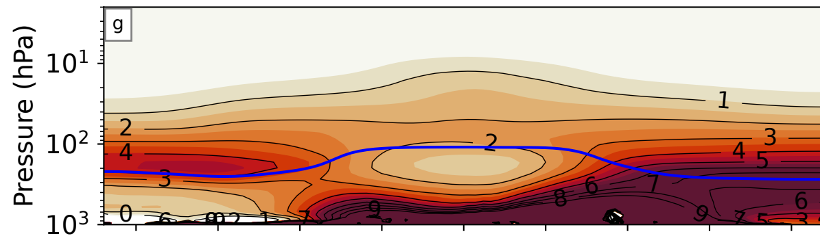
UM-UKCA
