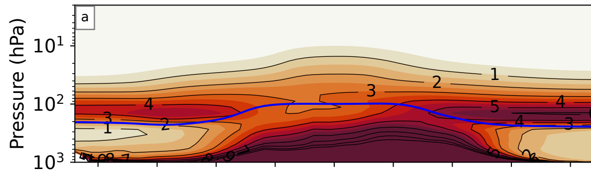
ECHAM6-SALSA
