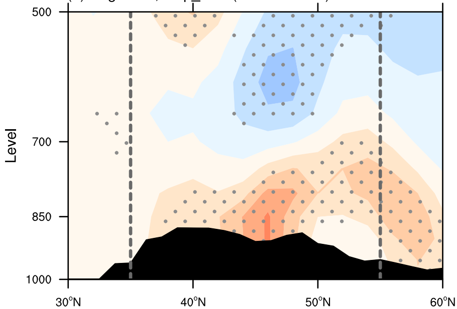
(b) Reg<Prec,temp_adv>(102.5-112.5E)
