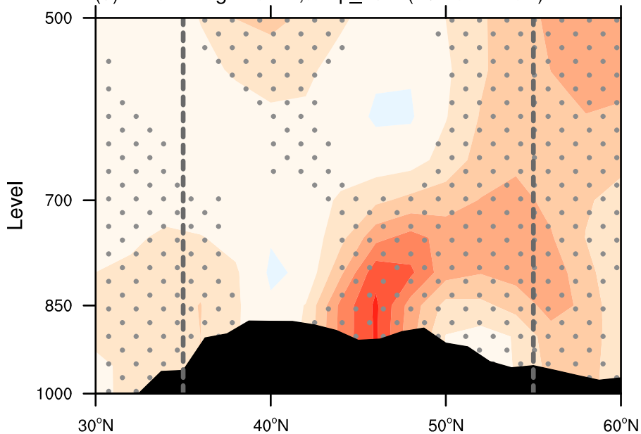
(d) Partial Reg<-IOBM,temp_adv>(102.5-112.5E)
