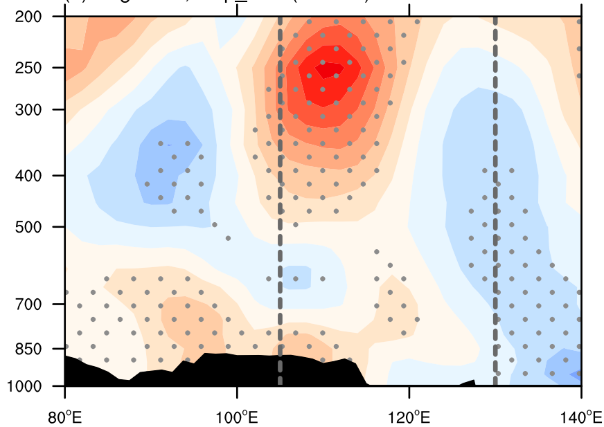
(a) Reg<Prec,temp_adv>(38-46N)
