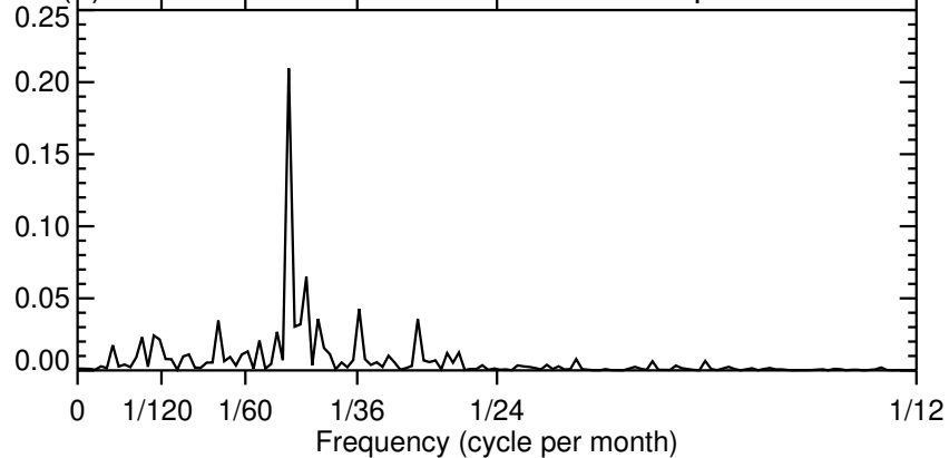
(d) PSD of stand. QNI from run 2 of Coupled-NINT-AP
