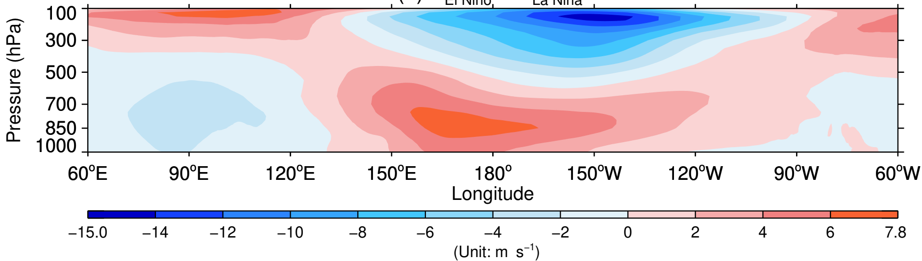
(c) \bar{u}_{\text{El Niño}} - \bar{u}_{\text{La Niña}}
