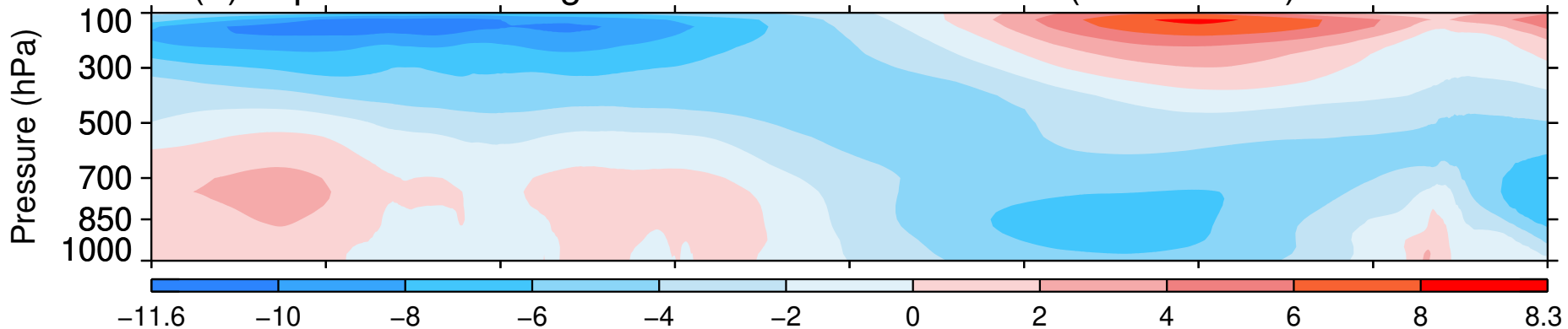
(c) \bar{u}_{\text{El Niño}} - \bar{u}_{\text{La Niña}}
