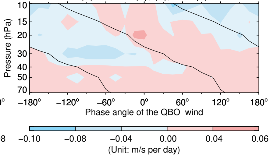
(d) Sum of (a), (b), and (c)
